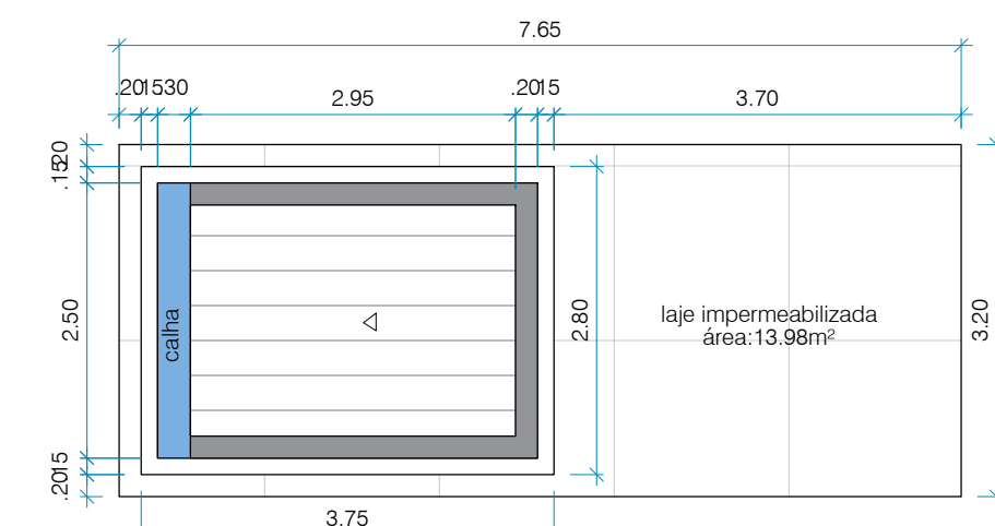
PLANTA DE COBERTA GUARITA ESCALA: 1/75
