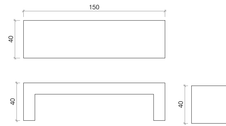
DETALHE BANCO BANCO DE CONCRETO ESC: 1/25
