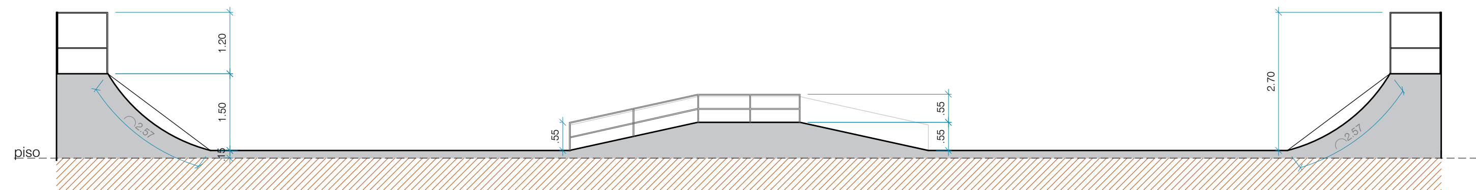
CORTE AA PISTA DE SKATE ESCALA: 1/100
