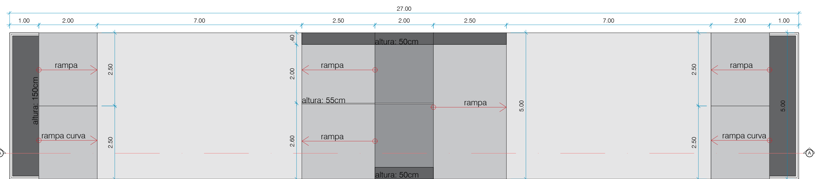
PLANTA BAIXA PISTA DE SKATE ESCALA: 1/100
