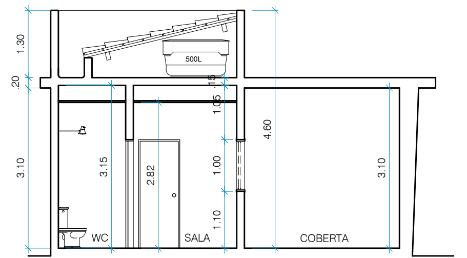
CORTE AA GUARITA ESCALA: 1/75
