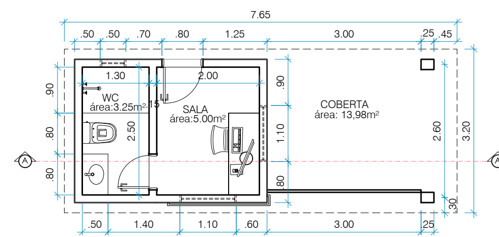
PLANTA BAIXA GUARITA ESCALA: 1/75
