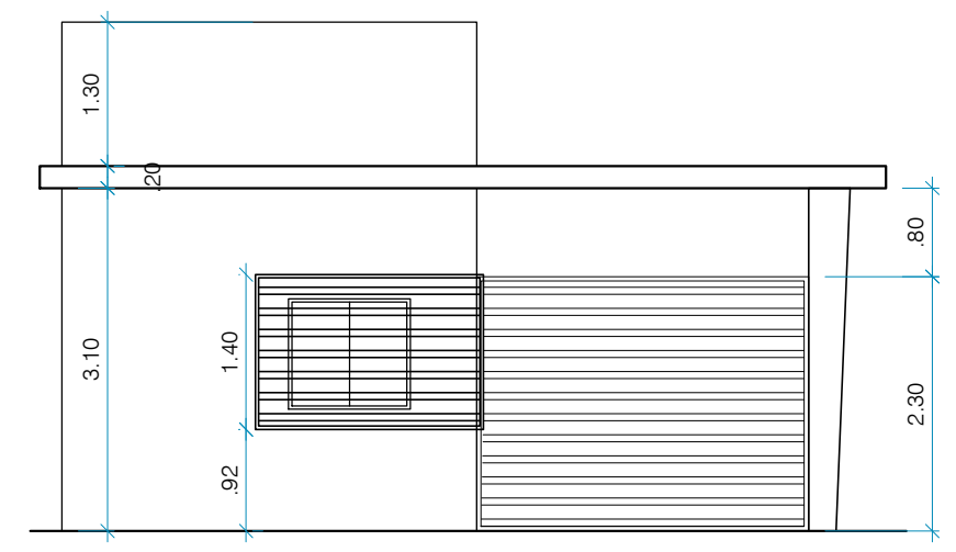
FACHADA SUDOESTE GUARITA ESCALA: 1/75
